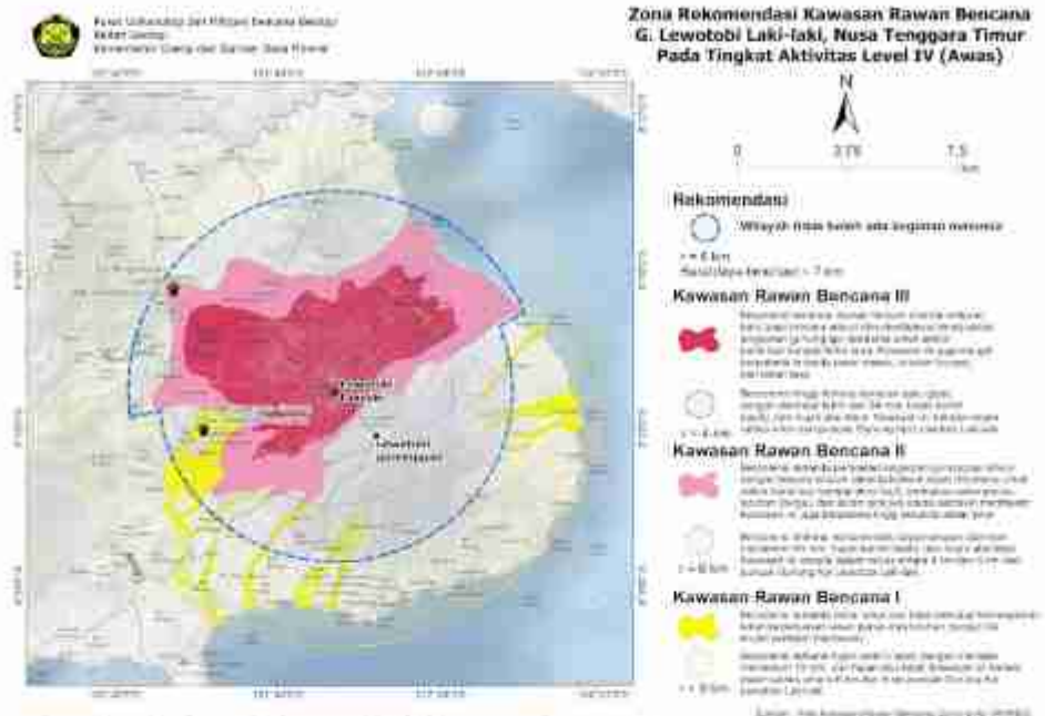
Gambar 2. Zona Rekomendasi Kawasan Rawan Bencana G. Lewotobi Laki-laki
