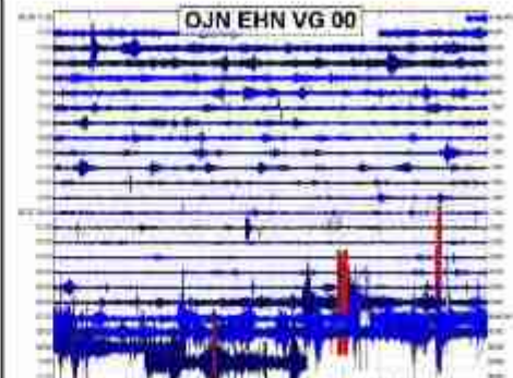
Gambar 6. Rekaman Seismik 24 Jam terakhir
