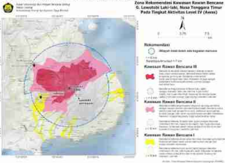
Gambar 8. Zona Rekomendasi Kawasan Rawan Bencana G. Lewotobi Laki-laki
