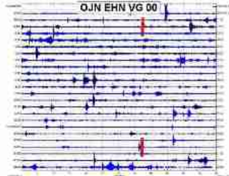
Gambar 4. Rekaman Seismik 24 jam terakhir.
