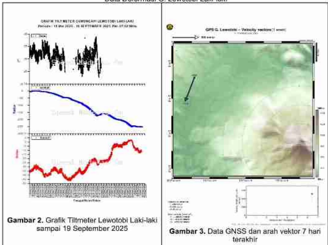
Data Deformasi G. Lewotobi Laki-laki
