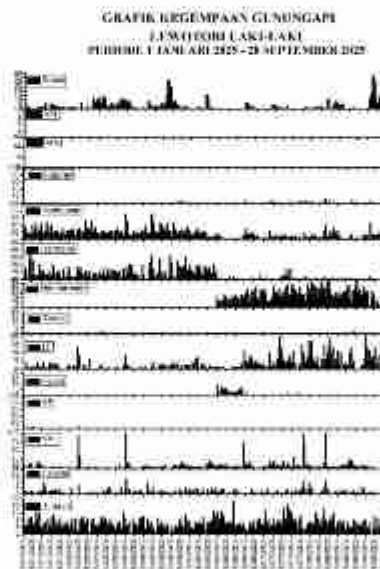
Gambar 5. Grafik Kegempaan 1 Januari 2025 - 28 September 2025
