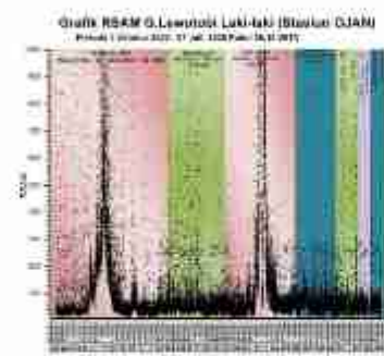
Gambar 4. Grafik Energi Seismik RSAM G. Lewotobi Laki-laki s.d. 7 Juli 2025
