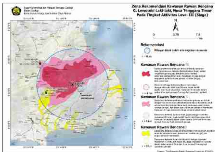
Gambar 8. Zona Rekomendasi Kawasan Rawan Bencana G. Lewotobi Laki-laki.
